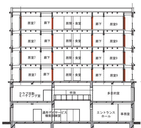
●断面図(東西) 0 1 2 3 (m)
