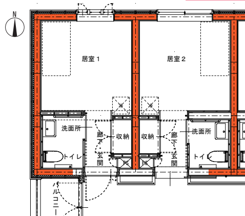
4-6階住戸平面詳細図
